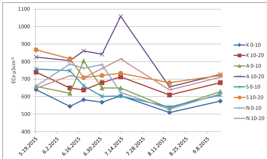
Joonis 4. Saku katseala erinevate katsevariantide (K – kontroll, A – adru 20 \text{ t ha}^{-1} , S – sõnnik 20 \text{ t ha}^{-1} ja N – NPK mineraalväetis 400 \text{ kg ha}^{-1} ) mulla soolsus 10 ja 20 cm sügavusel mullakihis
